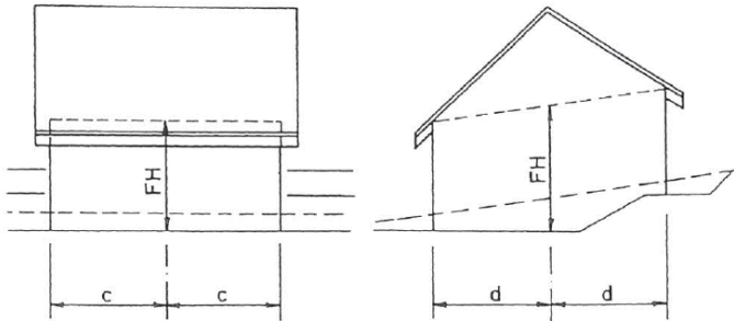
Fassadenhöhe bei Bauten am Hang
