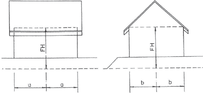
Fassadenhöhe bei Bauten am Hang
