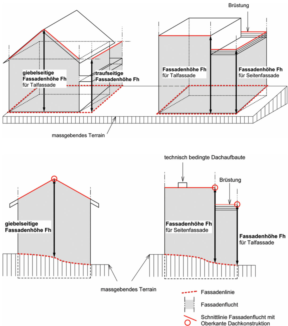
Figur 5.2 Gesamthöhe
