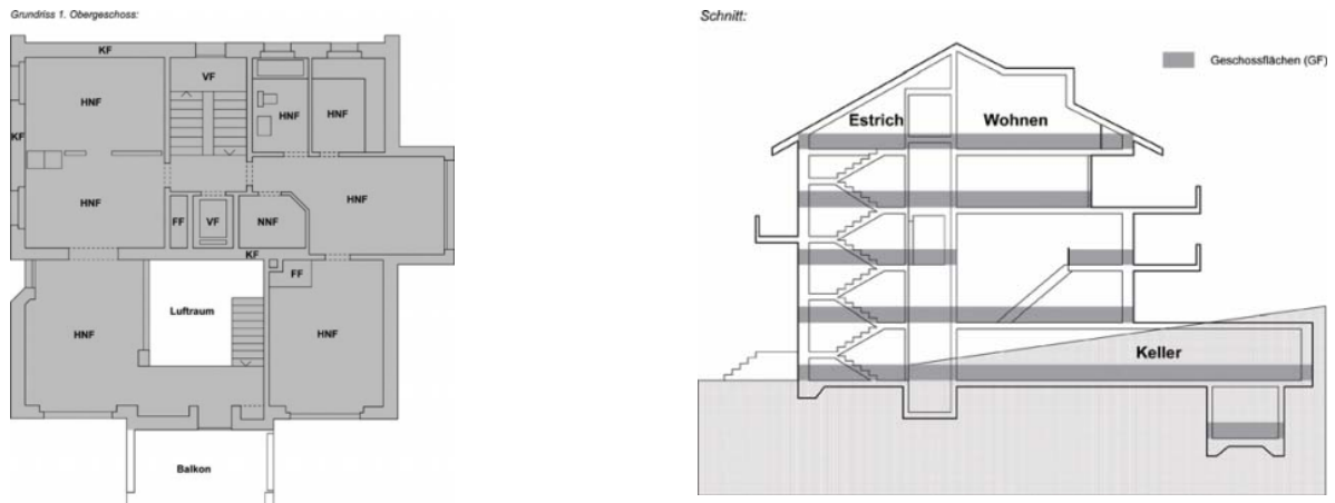
Figur 8.2 Geschossflächenziffer
