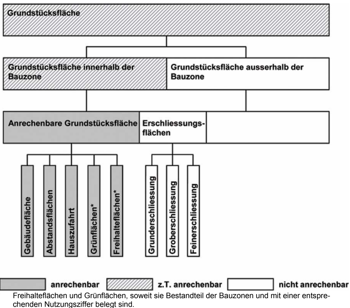
Figur 8.1 Anrechenbare Grundstücksfläche
