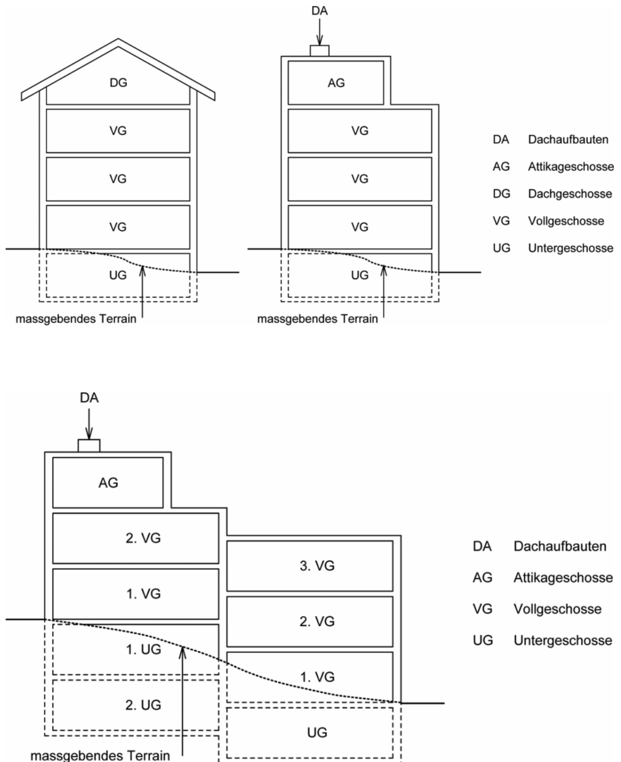
Figur 6.1 Geschosse und Geschosszahl
